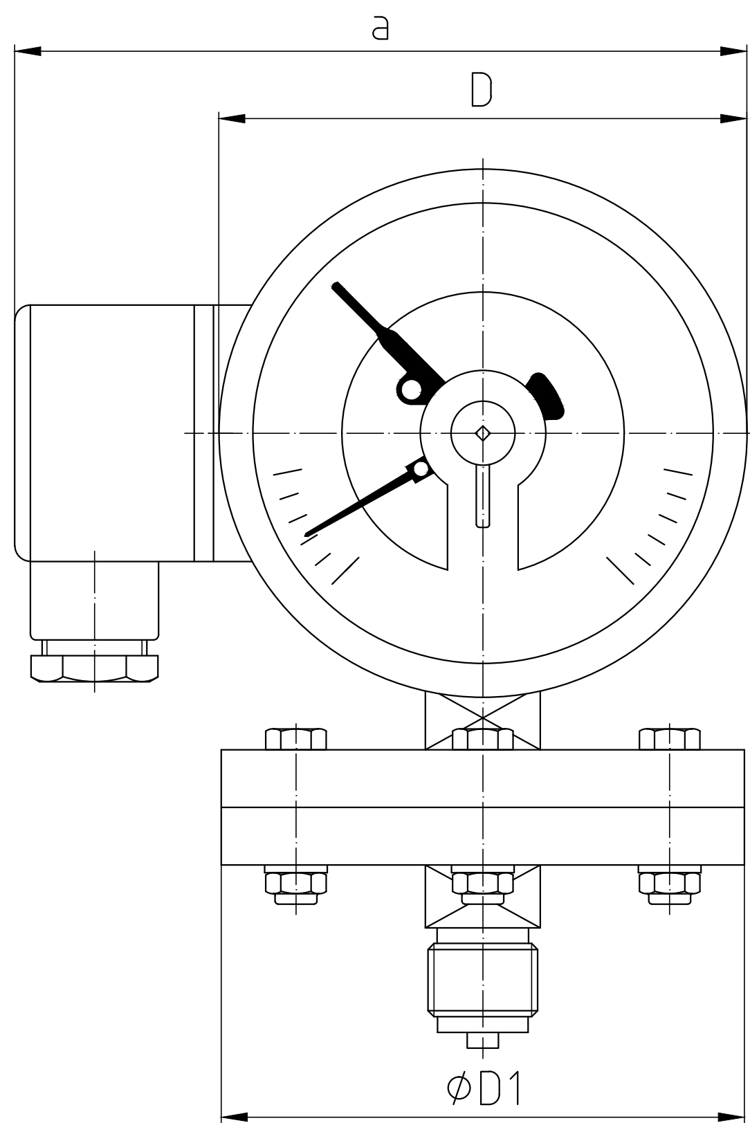
Fig. 140.10: mit Magnetspring- u. Schleichschaltung Fig. 140.20: mit Induktiv- u. Elektronikkontakt
